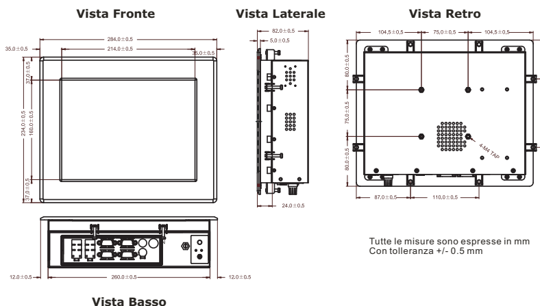
Disegno Meccanico
