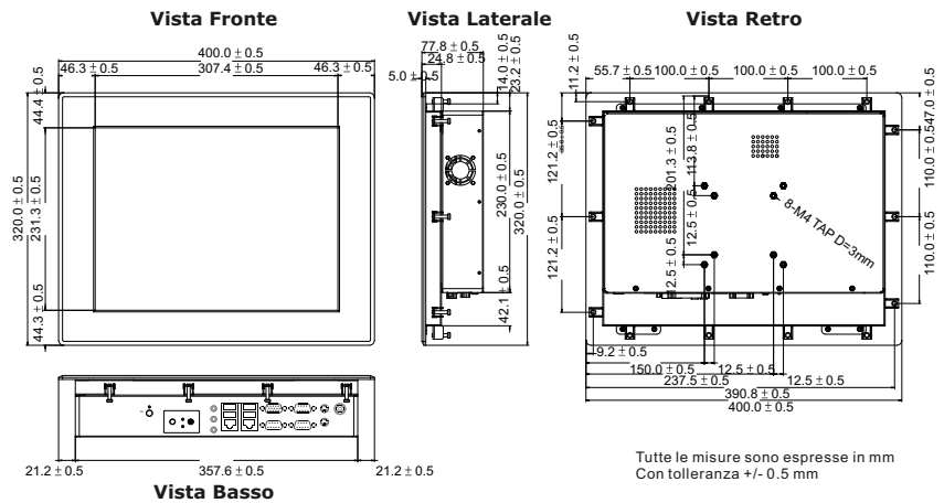
Disegno Meccanico
