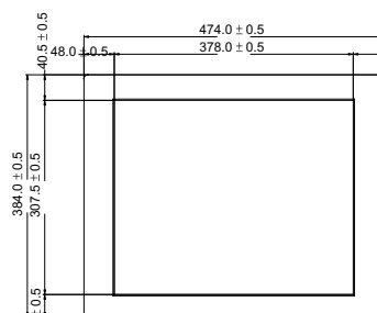
Vista Fronte
