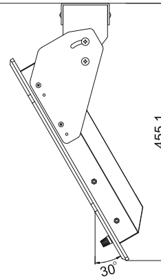
STAND ANGLE
