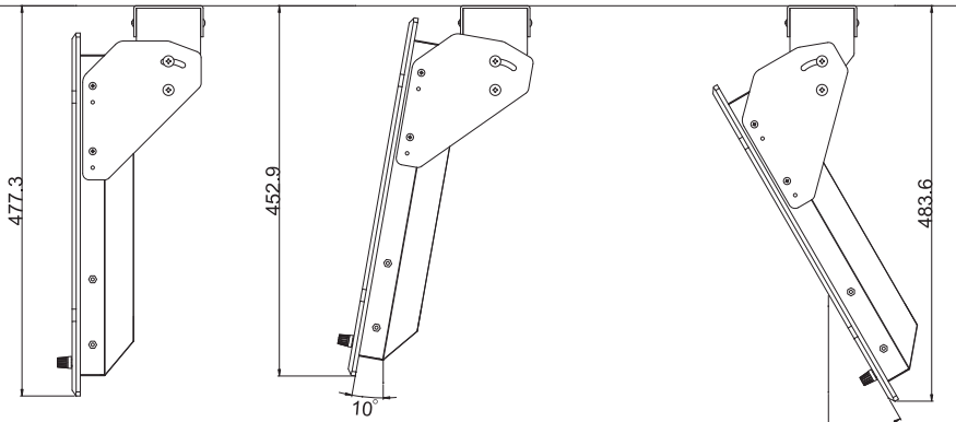
STAND ANGLE
