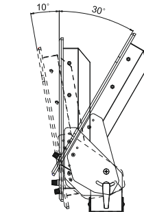
STAND ANGLE
