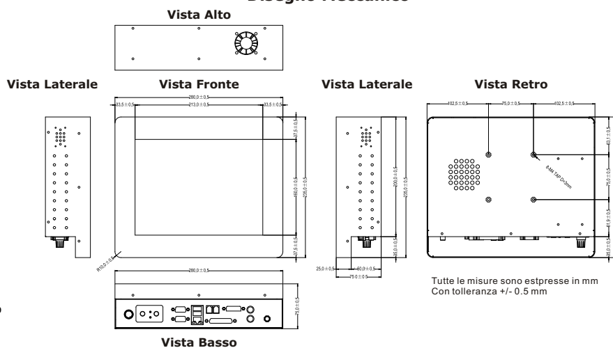
Disegno Meccanico
