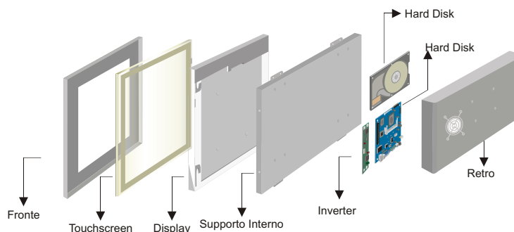
Disegno Meccanico
