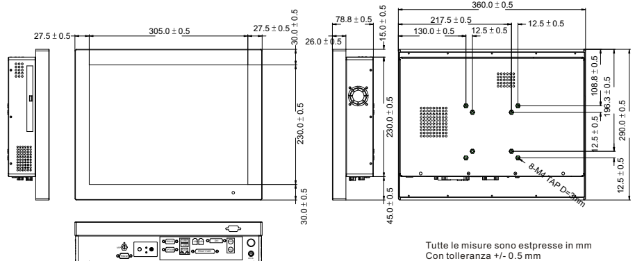
Vista Basso
