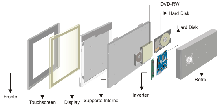
Disegno Meccanico
