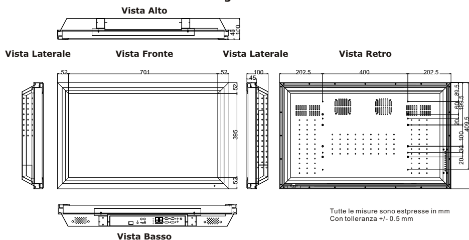
Disegno Meccanico
